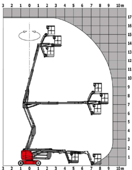
Braç articulat elèctric de 17m Manitou 170 AETJ-L
