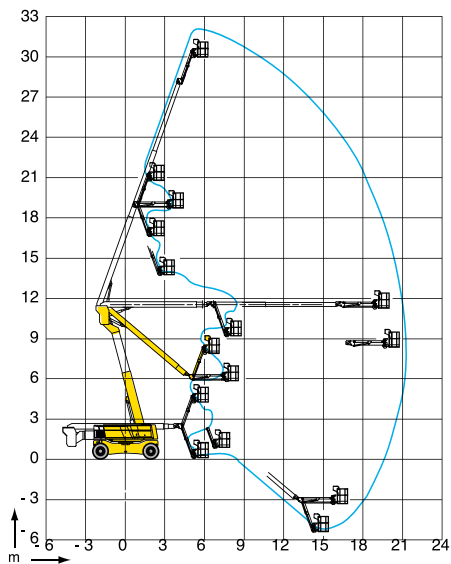
Braç articulat dièsel de 32m Haulotte HA32PX
