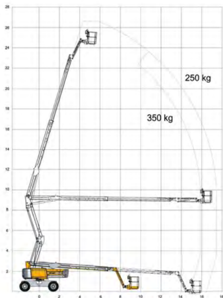
Braç articulat dièsel de 26m Haulotte HA26RTJ
