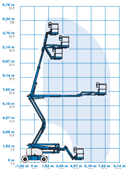
Braç articulat elèctric de 16m Genie Z4525J DC
