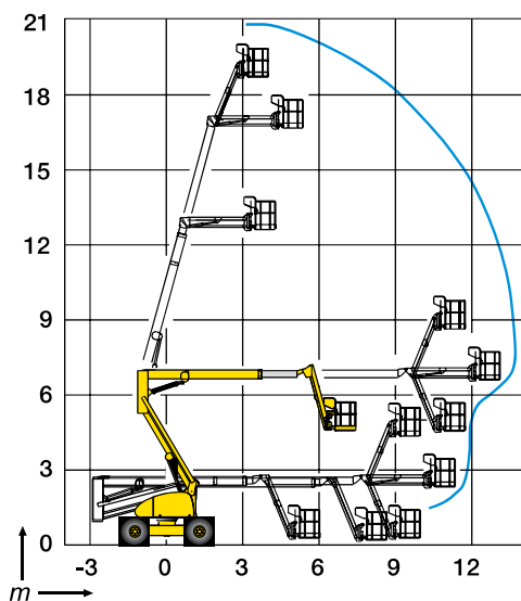
Braç articulat dièsel de 20m Haulotte HA20PX
