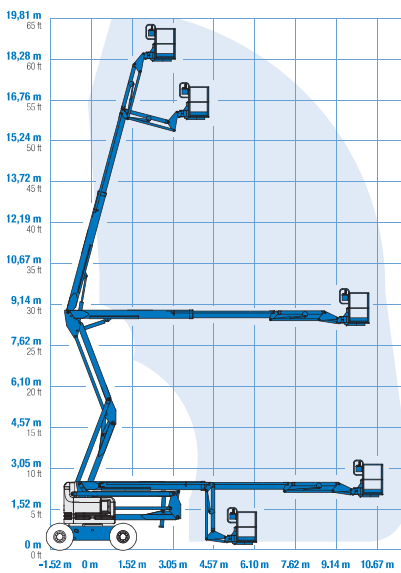
Braç articulat dièsel de 20m Genie Z6034
