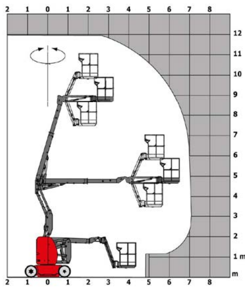
Braç articulat elèctric de 12m Manitou 120 AETJ
