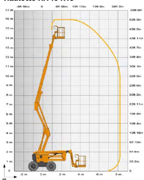
Braç articulat dièsel de 16m Haulotte HA 16 RTJ
