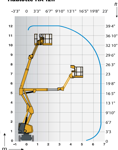
Braç articulat elèctric de 12m Haulotte HA 12IP
