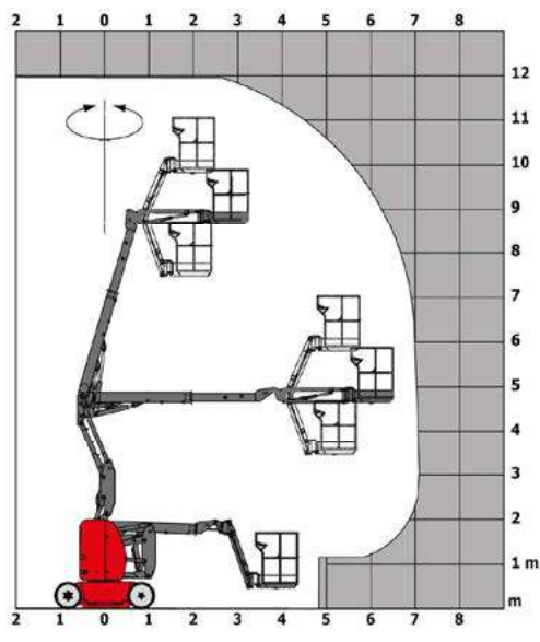
Braç articulat elèctric de 12m Manitou 120 AETJ
