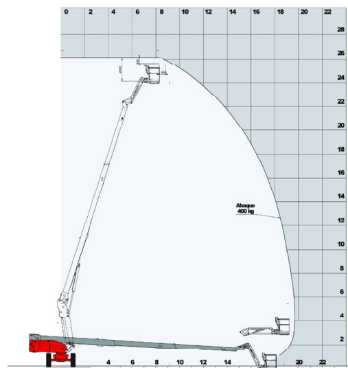
Braç telescòpic dièsel de 26m Manitou 260TJ
