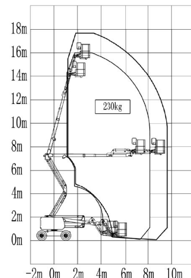
Braç articulat dièsel de 16m i 18m LGMG AR14J / LGMG AR16J
