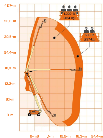
Braç articulats dièsel de 40m JLG 1250 AJP
