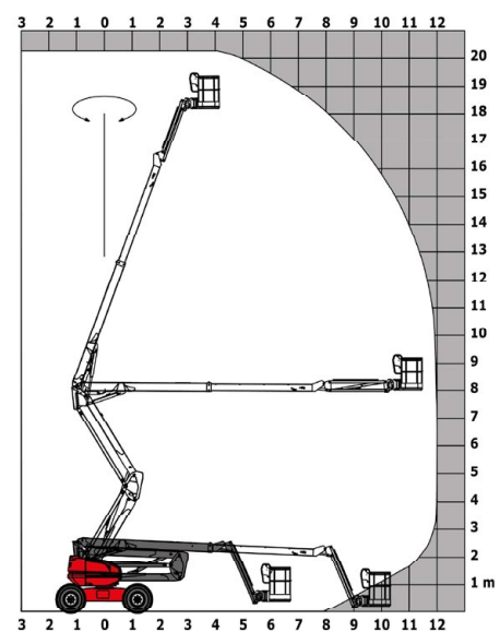
Braç articulat dièsel de 20m Manitou 200ATJ
