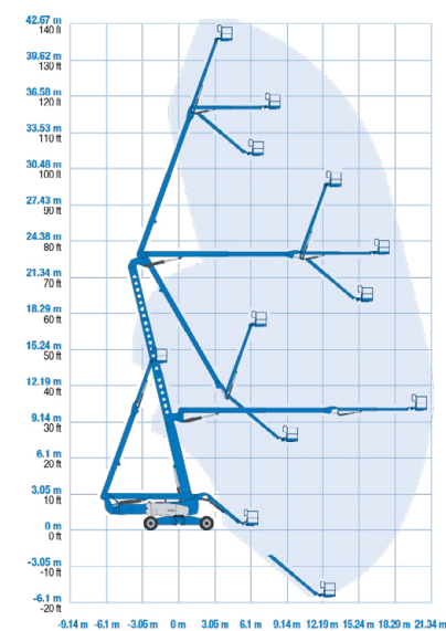
Braç articulats dièsel de 43m Genie Z135/70
