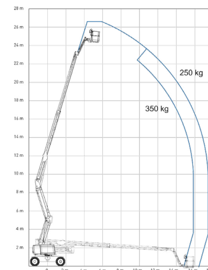
Braç articulats dièsel de 26m Haulotte HA 26RTJ
