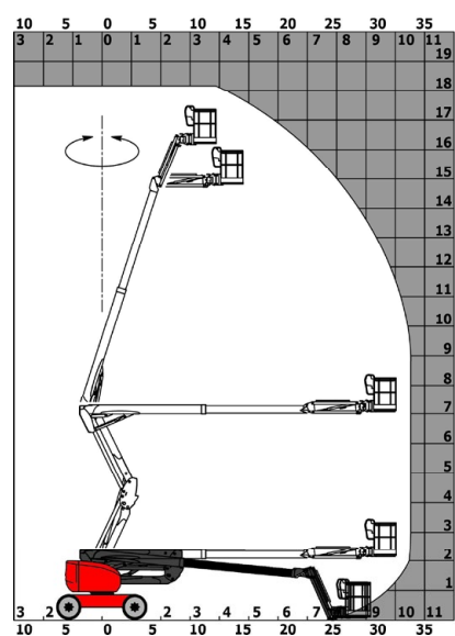
Braç articulat dièsel de 18m Manitou 180ATJ
