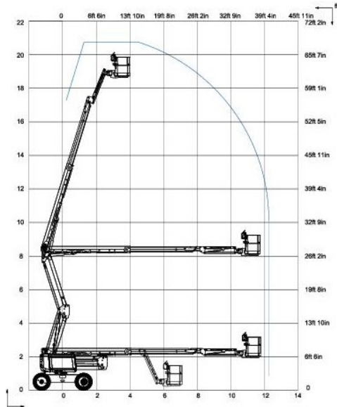
Braç articulat dièsel de 20m Haulotte HA20 RTJ PRO
