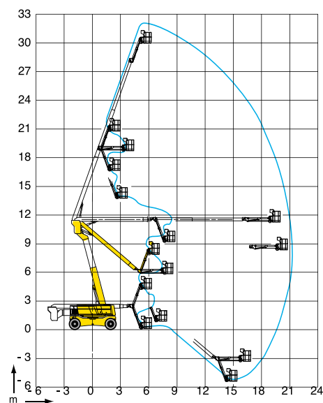
Braç articulats dièsel de 32m Haulotte HA 32PX
