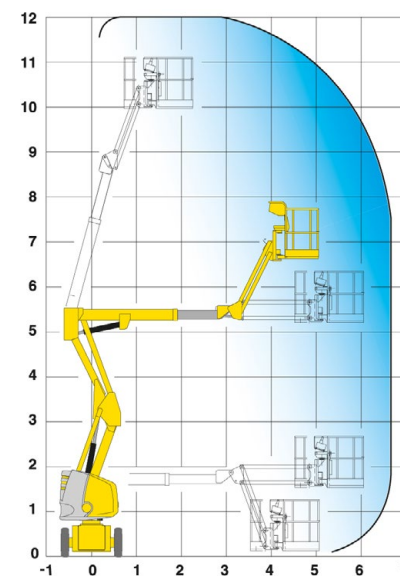
Braç articulat elèctric de 12m Haulotte HA 12IP
