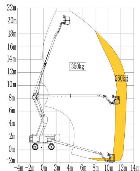
Braç articulat dièsel de 20m LGMG AR20J
