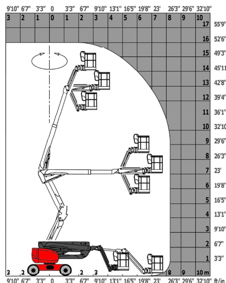
Braç articulat dièsel de 16m Manitou 160 ATJ
