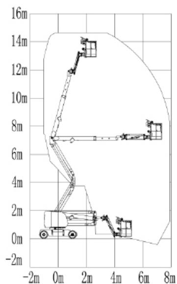
Braç articulat elèctric de 15m LGMG A13JE
