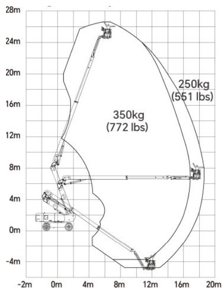
Braç articulats dièsel de 26m LGMG AR24J
