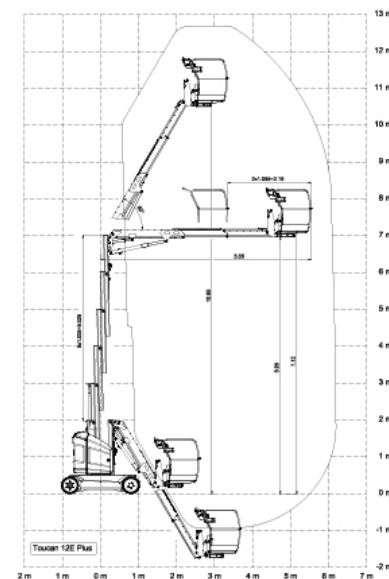
Braç articulat unipersonal de 12m JLG T12E- Plus
