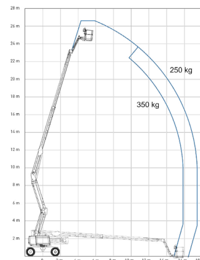
Braç telescòpic dièsel de 26m LGMG 26JH
