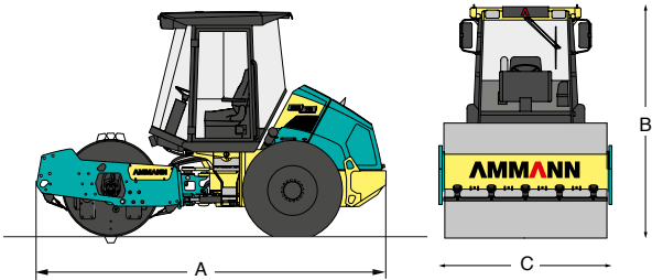
Compactadora ARS70
