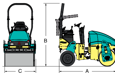
Compactadora ARX26
